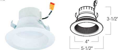
NLPR-442 Baffle
