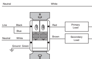
DSW-200 Bi-Level Wiring
