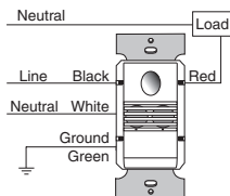
DSW-100 Wiring
